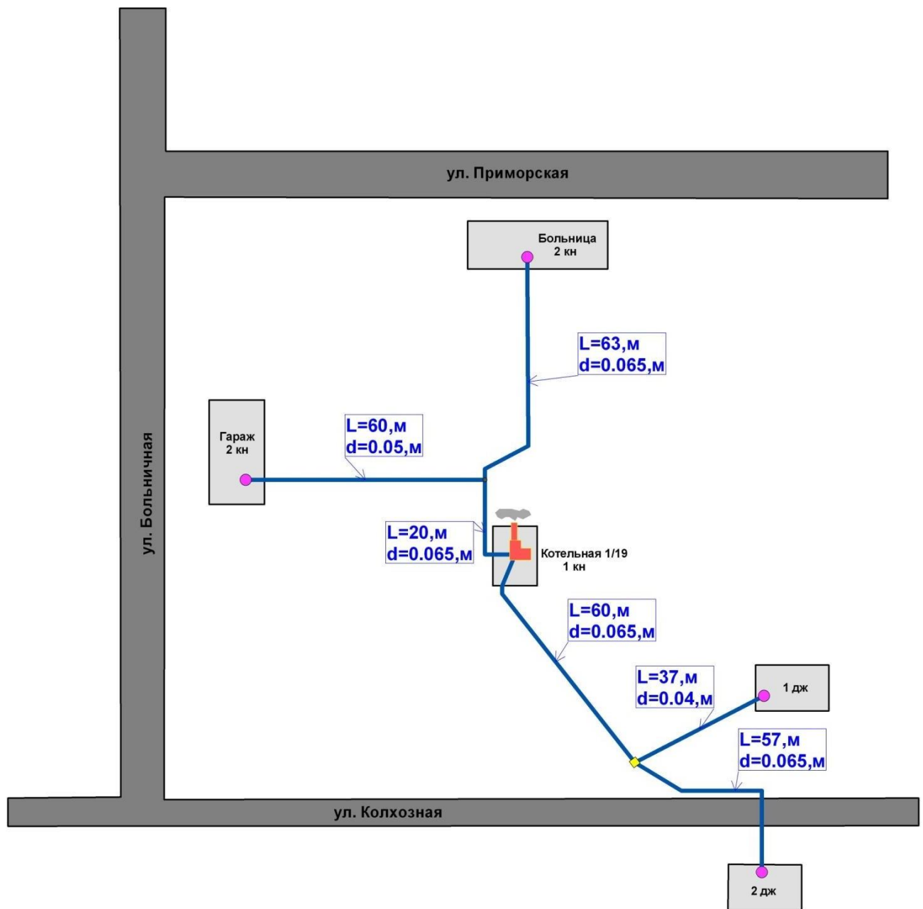
Рис. 2.2 – Схема теплоснабжения котельной АМК №1/19
