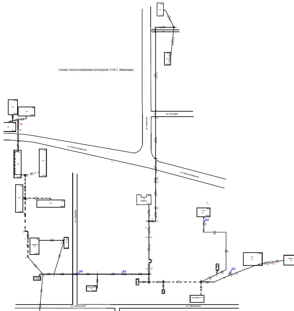
Рис. 2.1 – Схема теплоснабжения котельной №1/18
